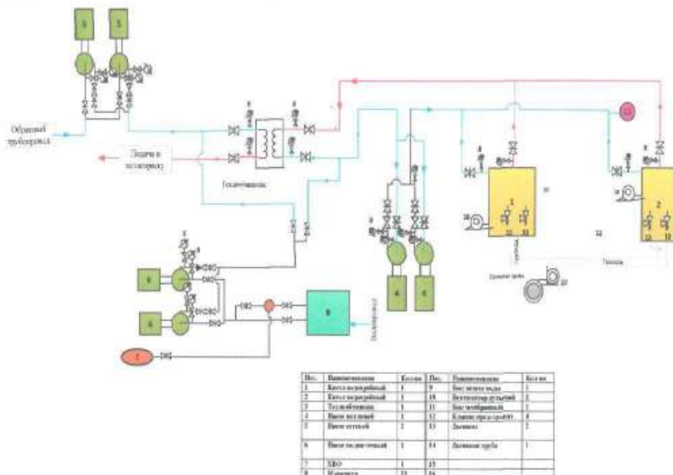
Рисунок 2.1 – Тепловая схема котельной с водогрейными котлами:
