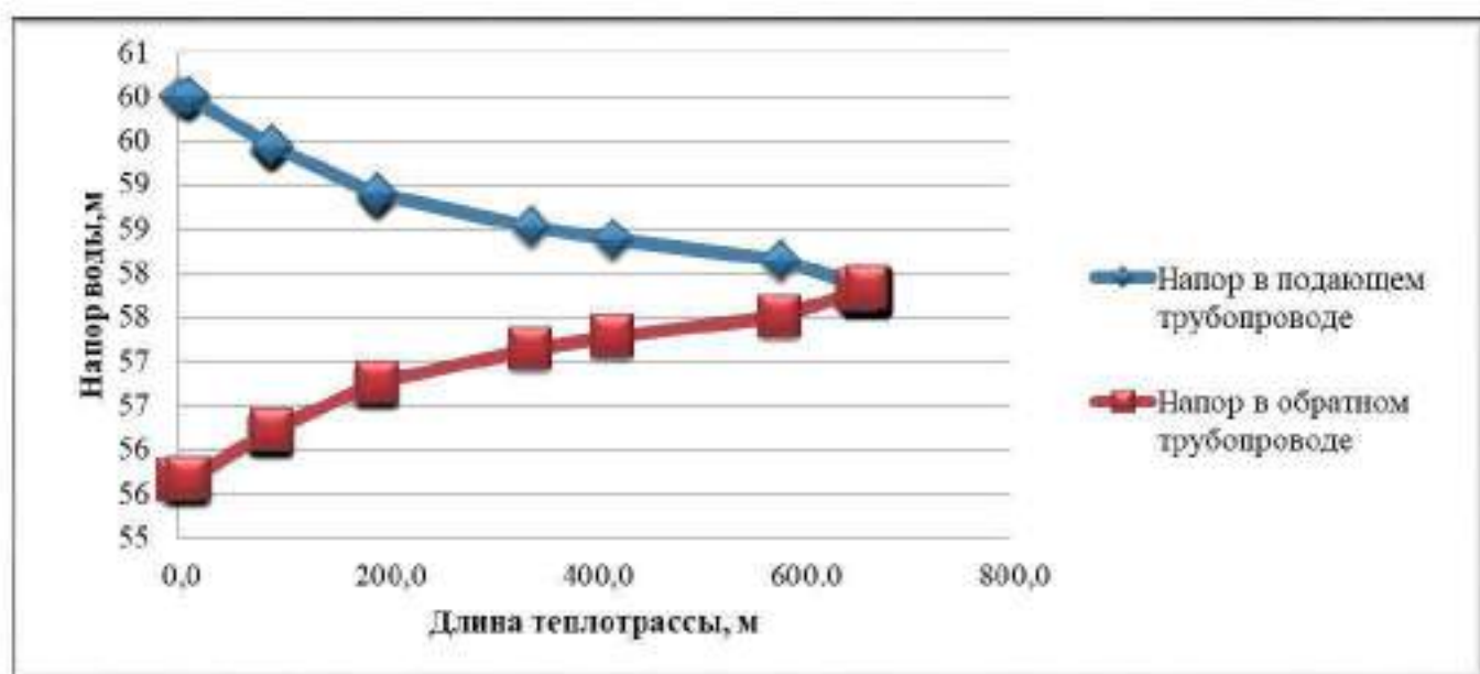
Рисунок 2.4 – Пьезометрический график тепловой сети котельной с. Боголюбовка по магистральному выводу от котельной до потребителя по переулку Школьный, 12
