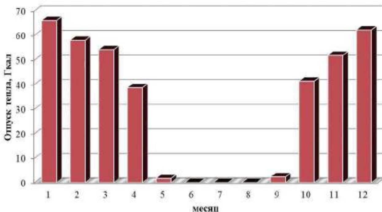
Рисунок 1.3 – Оптимальный температурный график отпуски тепловой энергии для котельной д. Большая Рошка
