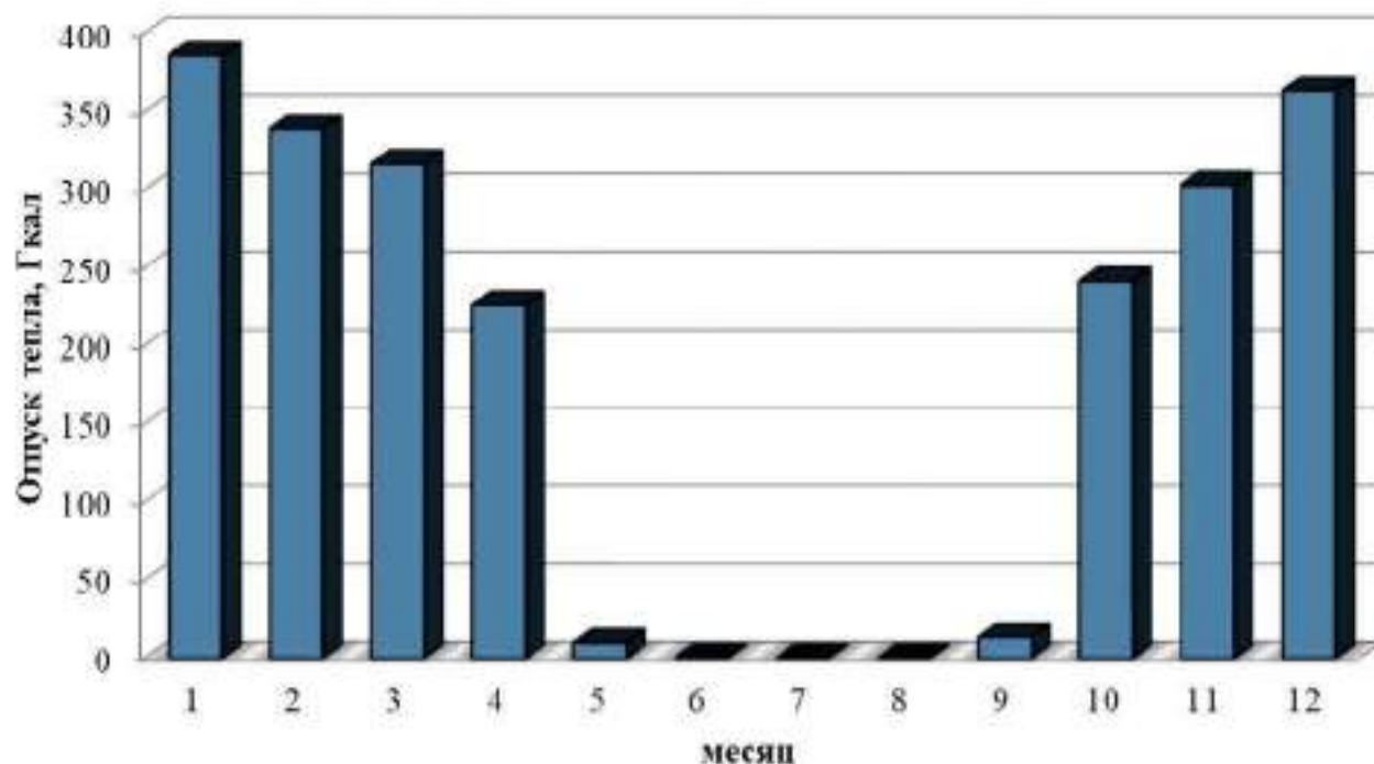
Рисунок 1.2 – Оптимальный температурный график отпуски тепловой энергии для котельной с. Боголюбовка
