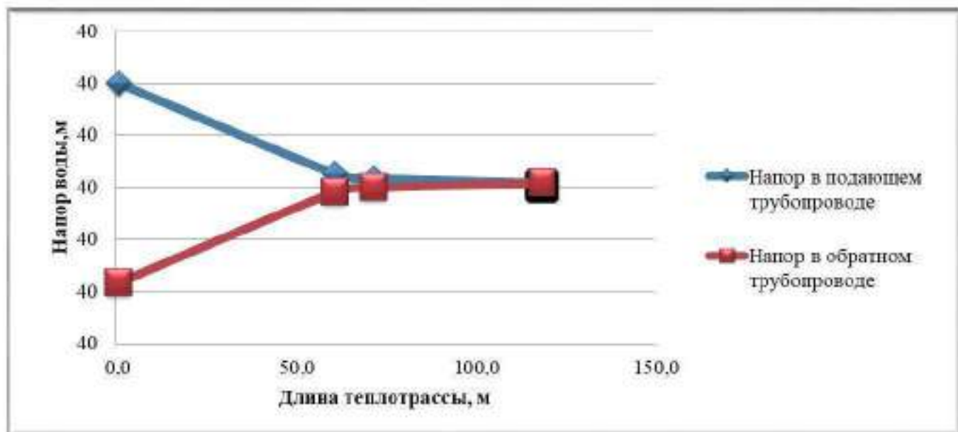
Рисунок 2.5 – Пьезометрический график тепловой сети котельной д. Большая Роща по магистральному выводу
