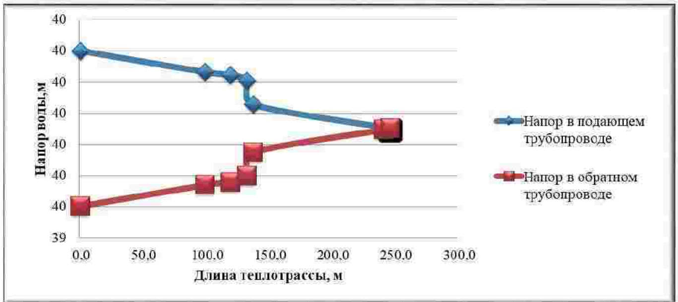
Рисунок 2.4 – Пьезометрический график тепловой сети котельной №2 по магистральному выводу
