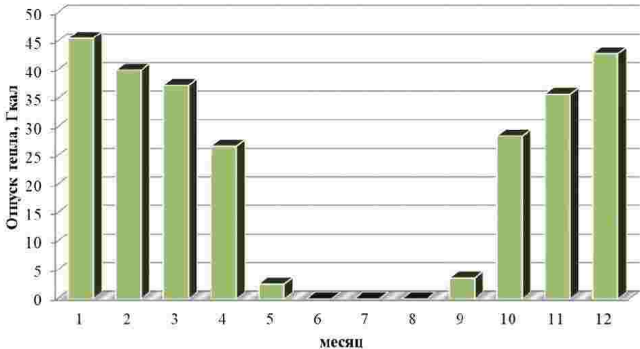
Рисунок 1.4 – Оптимальный температурный график отпуски тепловой энергии для котельной Березовской школы
