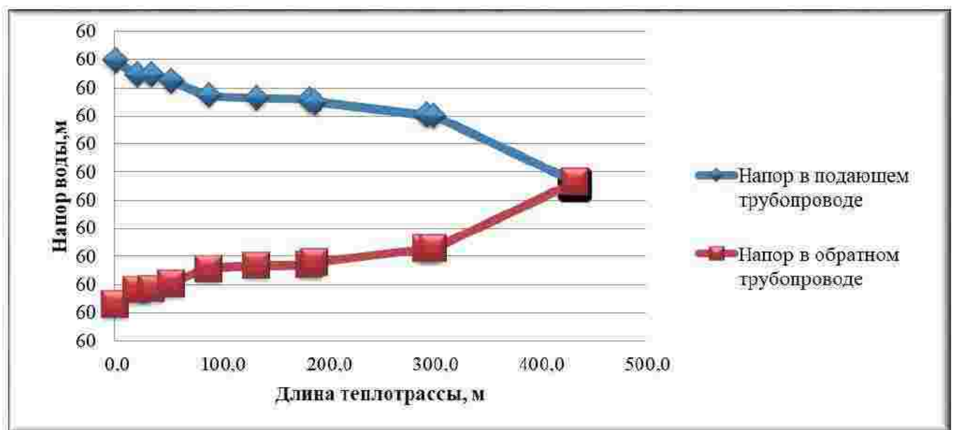
Рисунок 2.3 – Пьезометрический график тепловой сети котельной №1 по магистральному выводу
