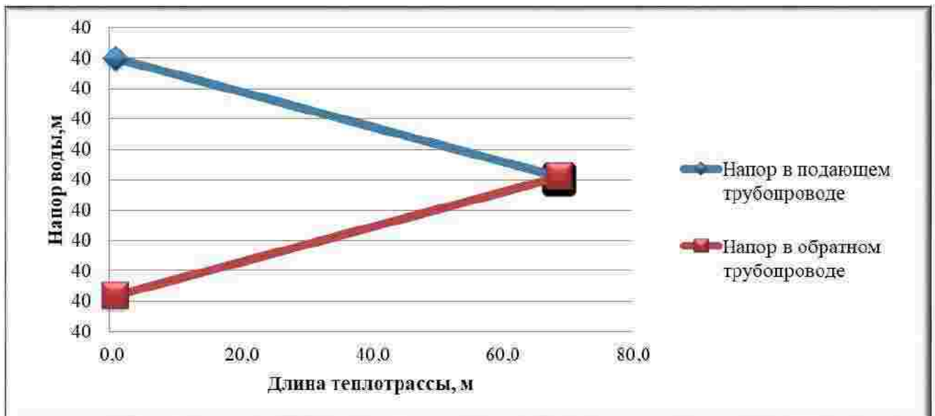
Рисунок 2.5 – Пьезометрический график тепловой сети котельной Березовской школы по магистральному выводу
