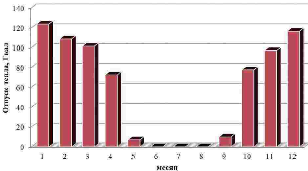
Рисунок 1.3 – Оптимальный температурный график отпуса тепловой энергии для котельной №2
