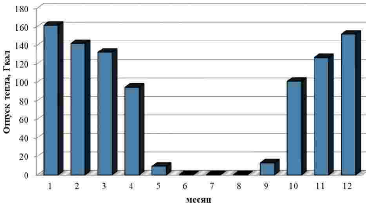
Рисунок 1.2 – Оптимальный температурный график отпуса тепловой энергии для котельной №1
