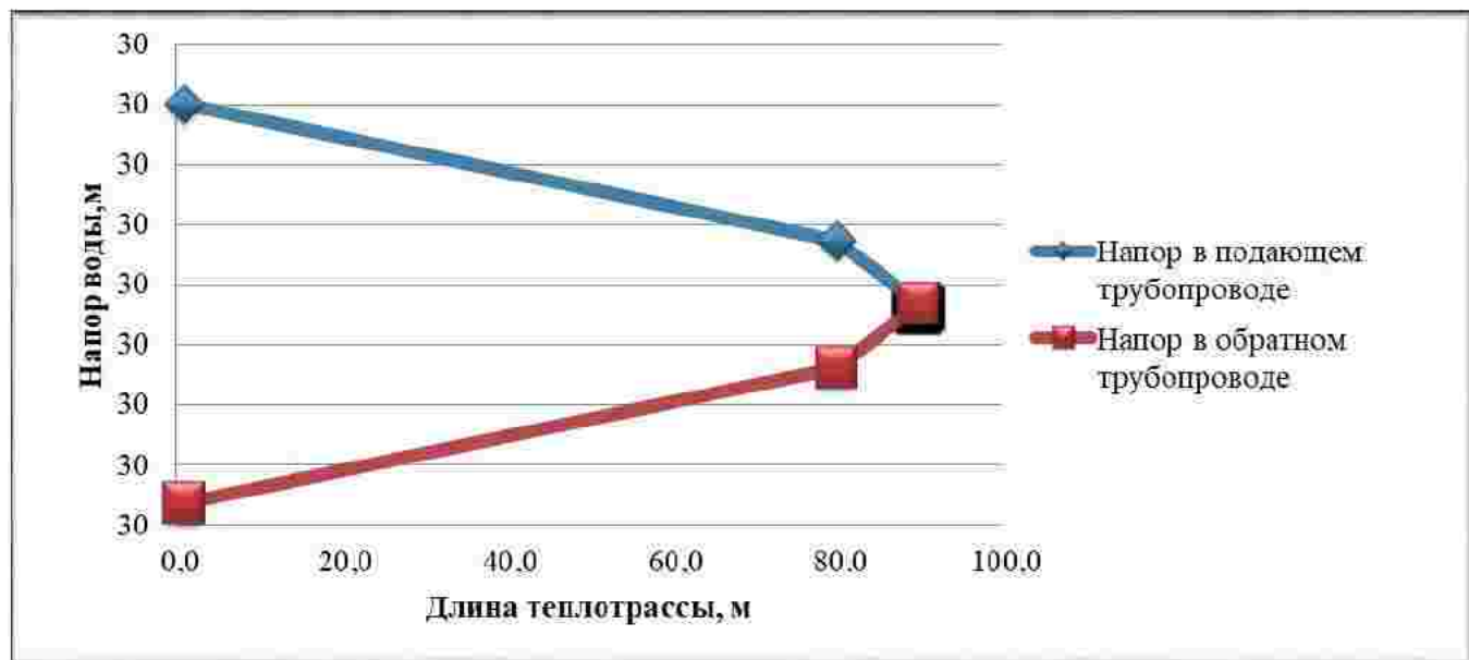
Рисунок 2.5 – Пьезометрический график тепловой сети котельной Администрации по магистральному выводу
