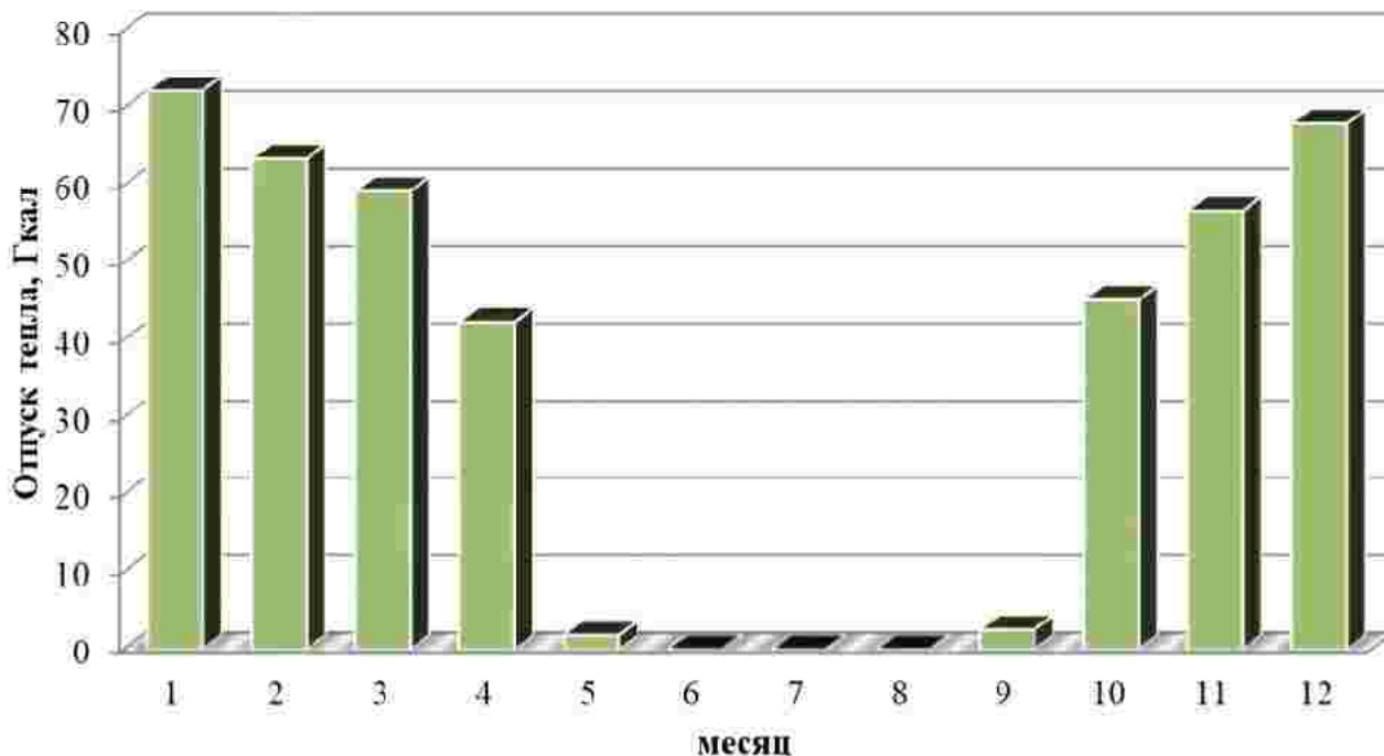
Рисунок 1.4 – Оптимальный температурный график отпуски тепловой энергии для котельной Администрации
