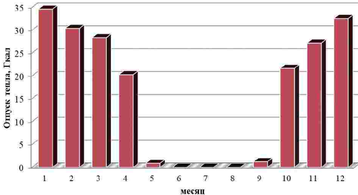
Рисунок 1.3 – Оптимальный температурный график отпуски тепловой энергии для котельной Детского сада
