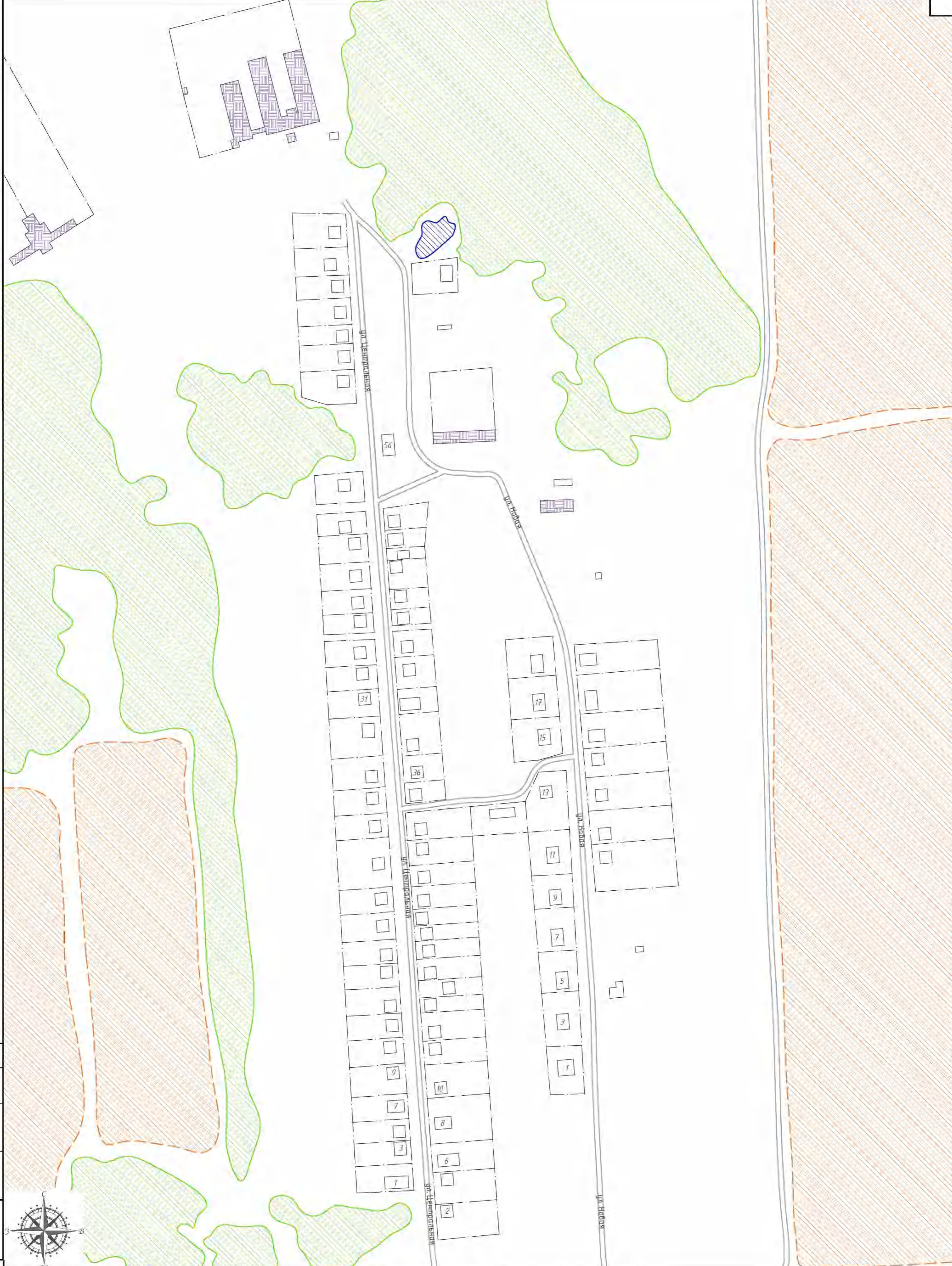
Условные обозначения
