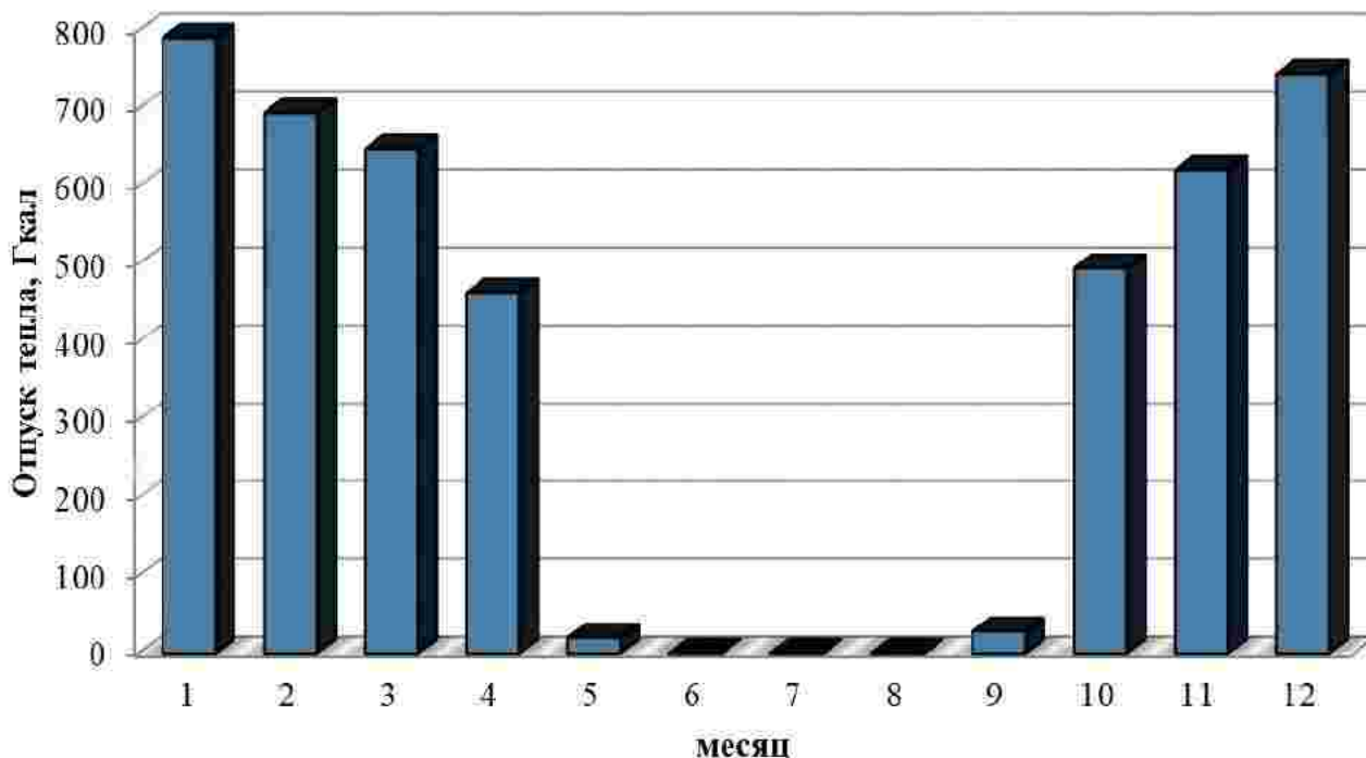
Рисунок 1.2 – Оптимальный температурный график отпуска тепловой энергии для котельной с. Степное
