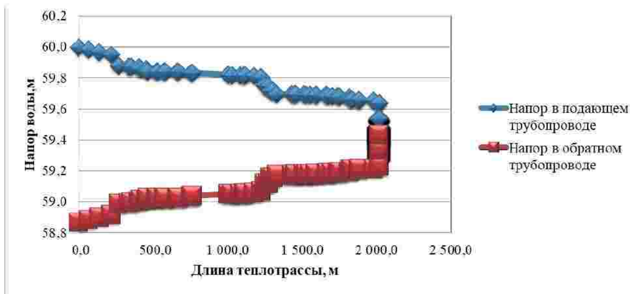
Рисунок 2.3 – Пьезометрический график тепловой сети котельной с. Степное по магистральному выводу
