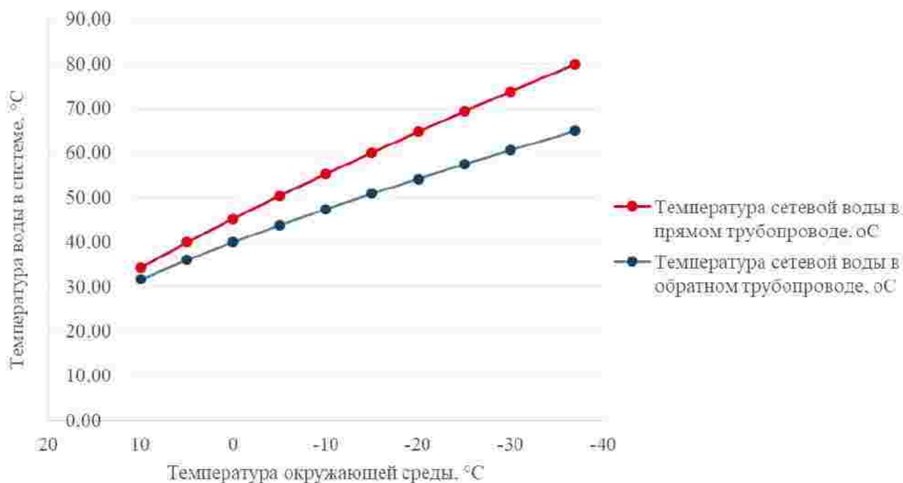
Рисунок 2.2 – График изменения температур теплоносителя (температурный график 80/65^{\circ}\text{C} )
