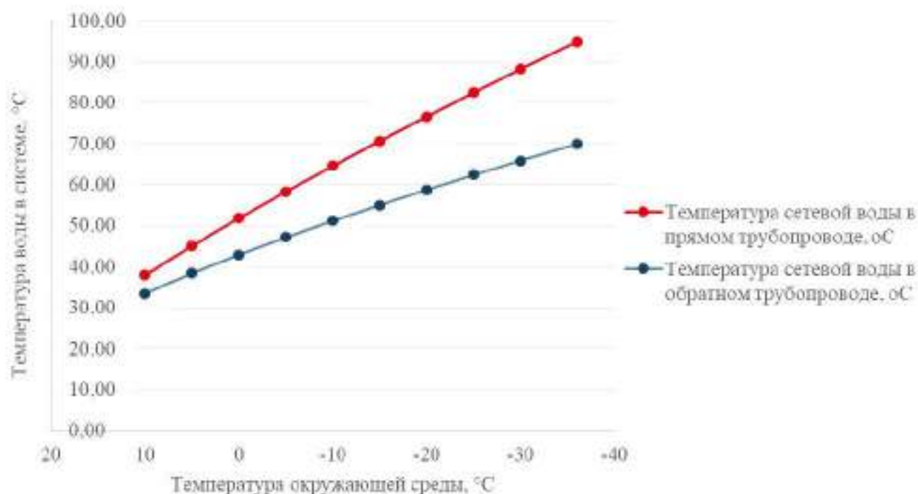
Рисунок 2.2 – График изменения температур теплоносителя (температурный график 95/70°C)
