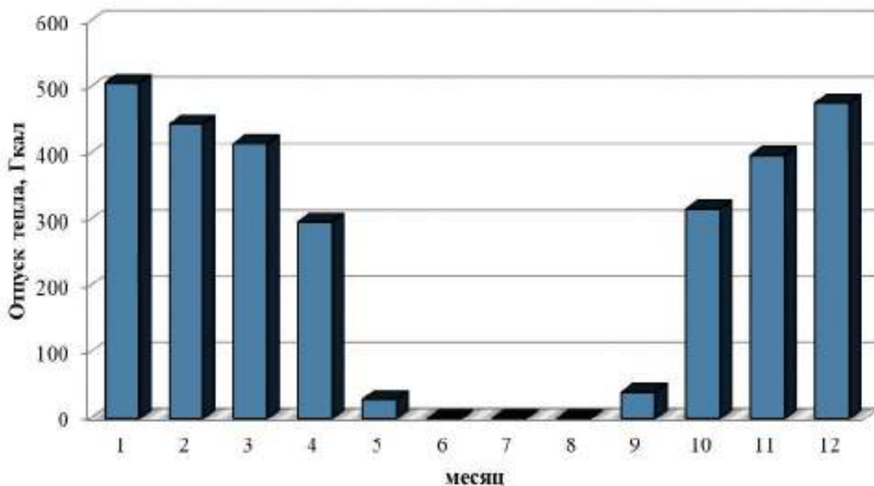
Рисунок 1.2 – Оптимальный температурный график отпуски тепловой энергии для котельной п. Конезаводский
