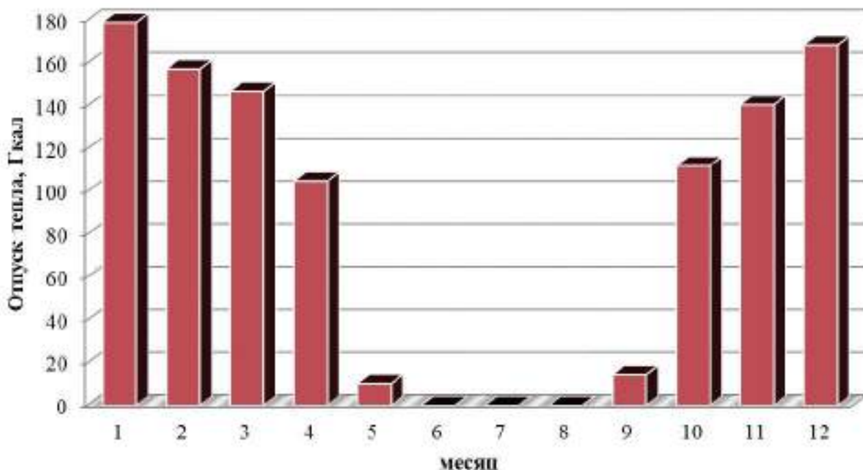
Рисунок 1.3 – Оптимальный температурный график отпуски тепловой энергии для котельной д. Васильевка
