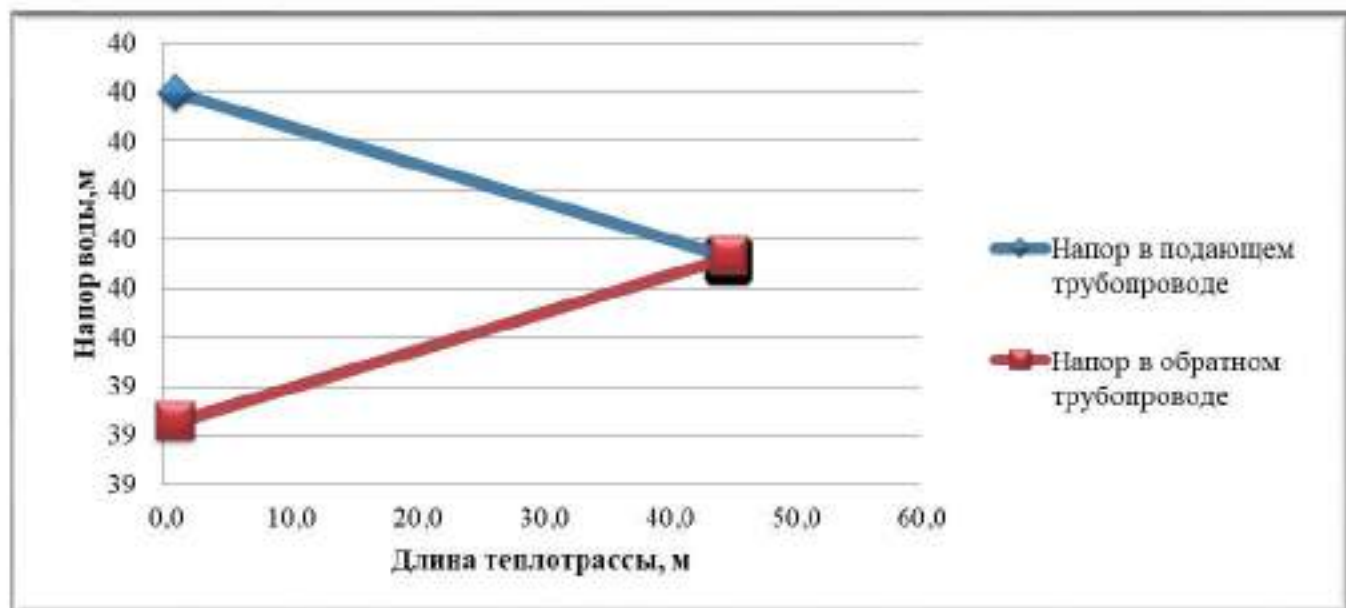
Рисунок 2.5 – Пьезометрический график тепловой сети котельной Алексеевской школы по магистральному выводу
