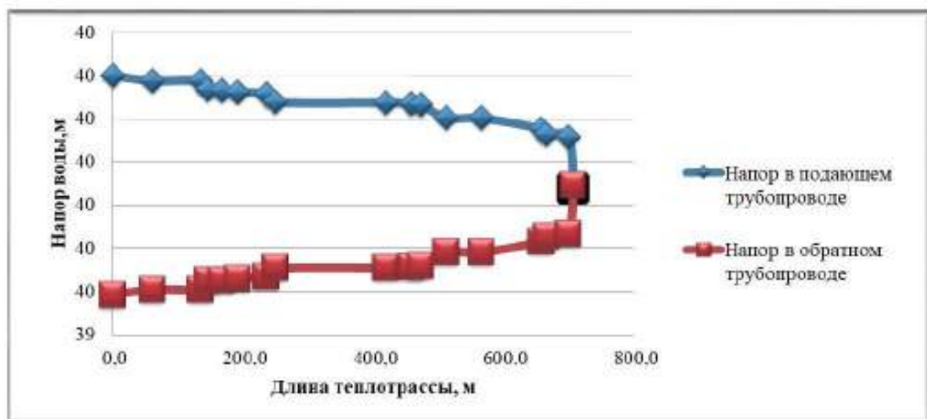
Рисунок 2.4 – Пьезометрический график тепловой сети котельной д. Васильевка по магистральному выводу
