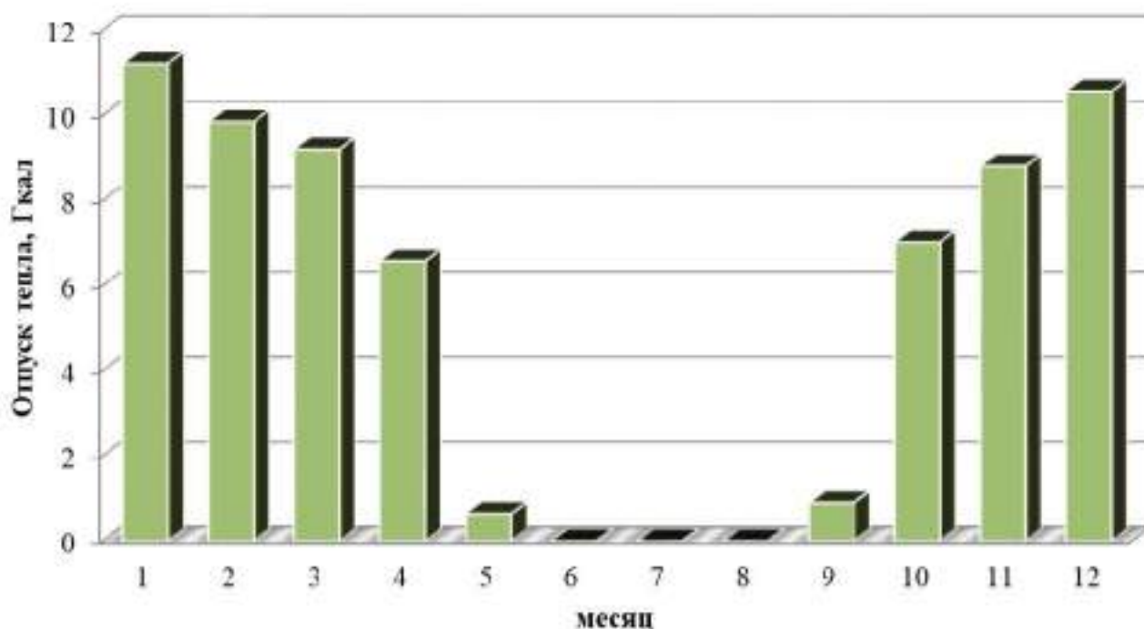
Рисунок 1.4 – Оптимальный температурный график отпуски тепловой энергии для котельной Алексеевской школы
