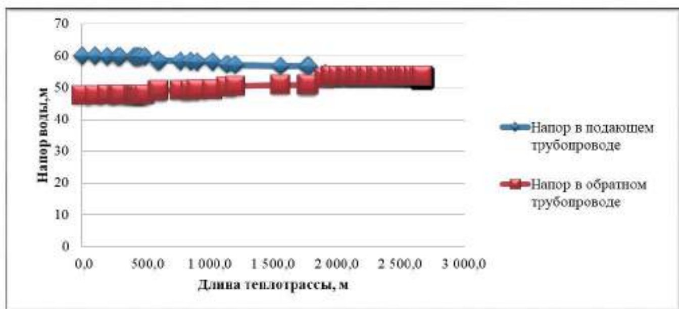
Рисунок 2.3 – Пьезометрический график тепловой сети котельной п. Конезаводский по магистральному выводу
